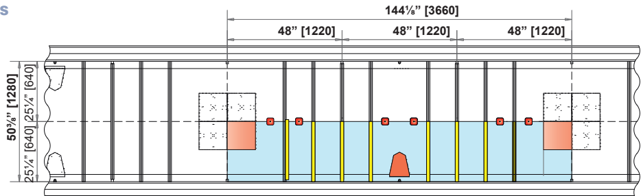
Cestón Cage 144 1/8" x 25 1/4" [3660 x 640] - 30 aves pondeuses
